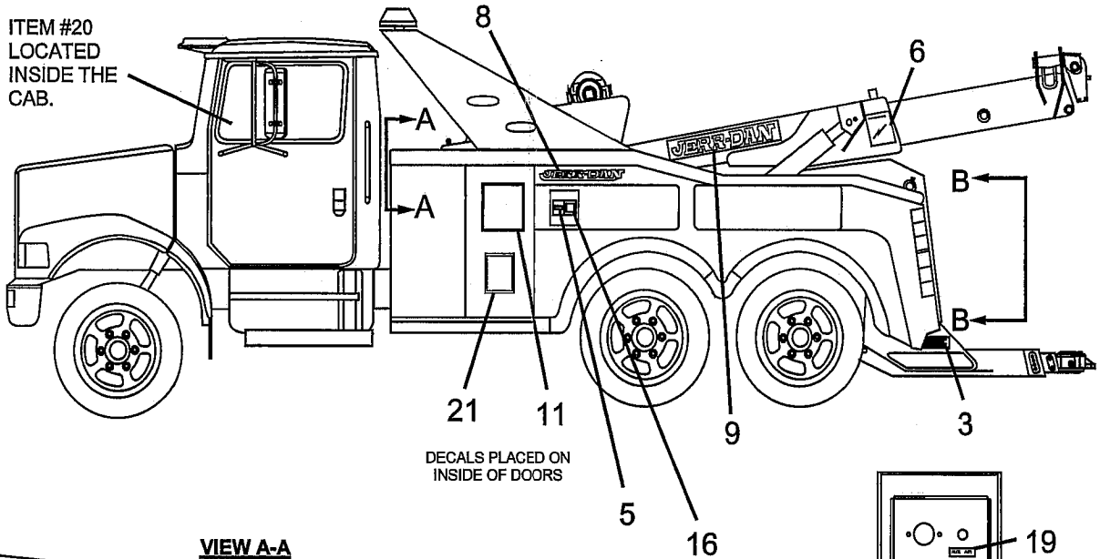
VIEW A-A
