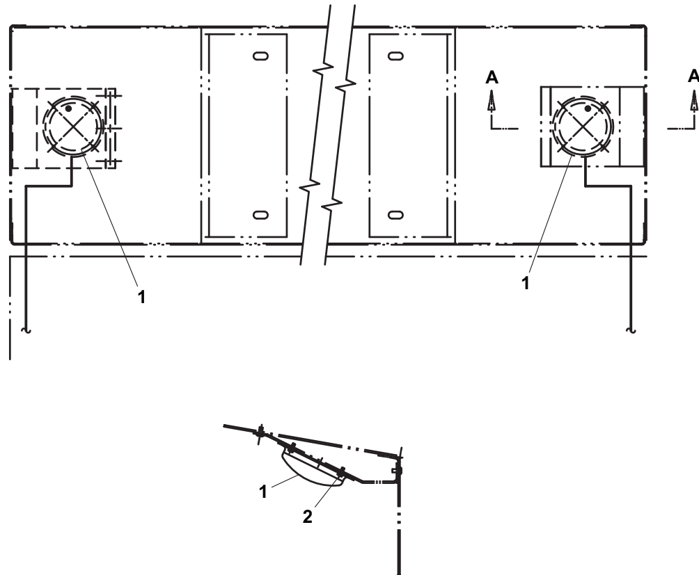
VIEW A-A
